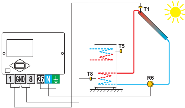
Bild 1- Brauchwassererwärmer
