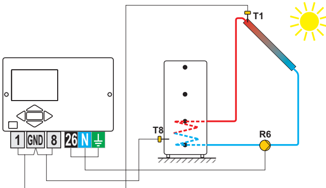
Bild 2- Wärmespeicher
